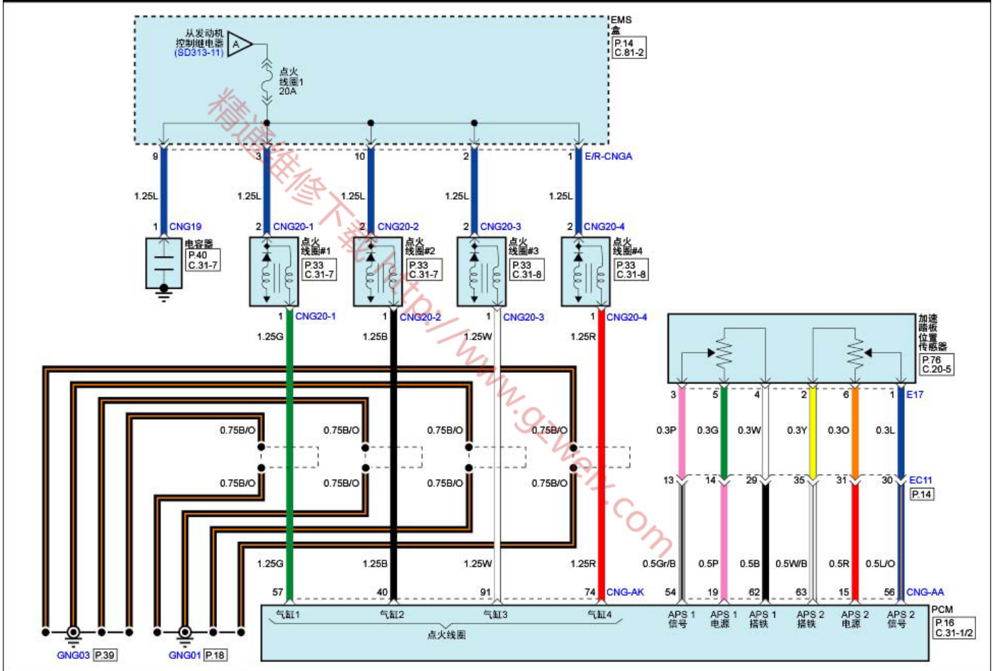
发动机控制系统(G4NB : NU 1.8L MPI A/T)(6)
